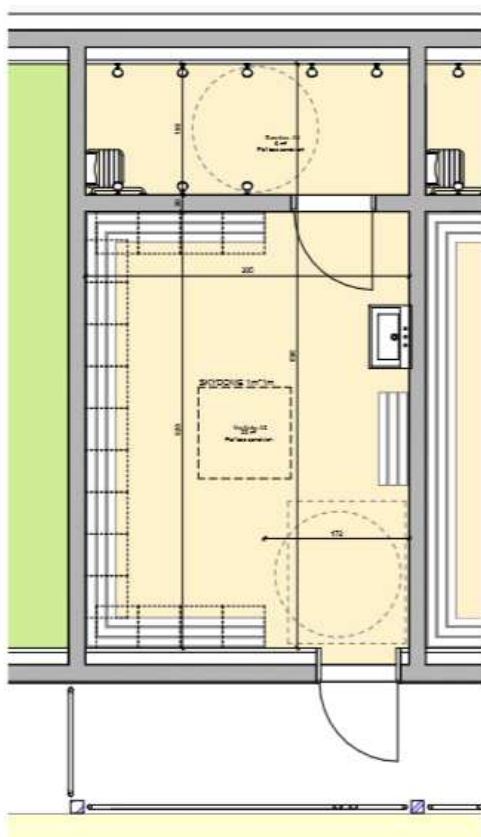
Aménagement type vestiaires
